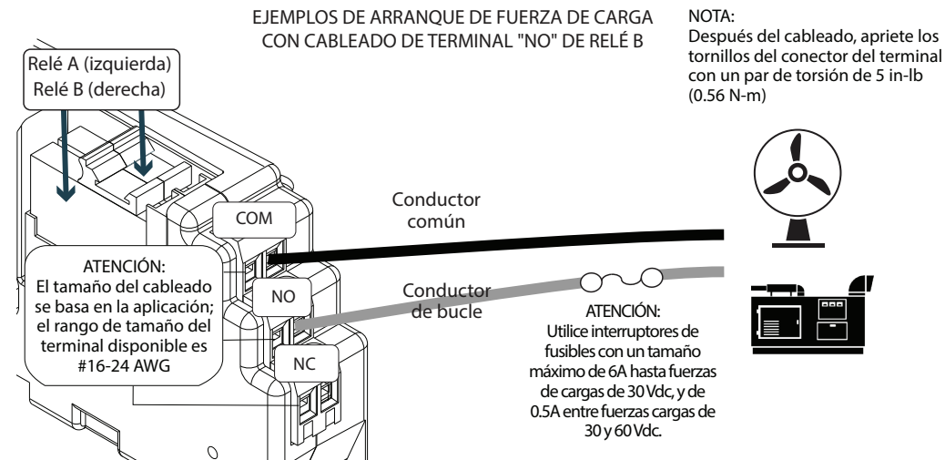
Figura 5-1 - Detalle del arranque de la fuerza de carga
