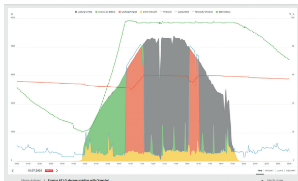
Bilancio energetico giornaliero
