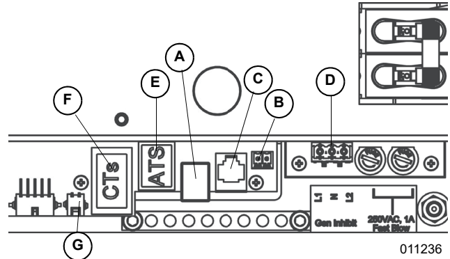
Figura 5-10. Puertos auxiliares
