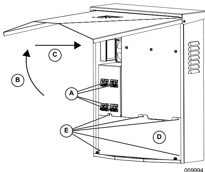
Figura 7-1. Compartimiento de cableado
