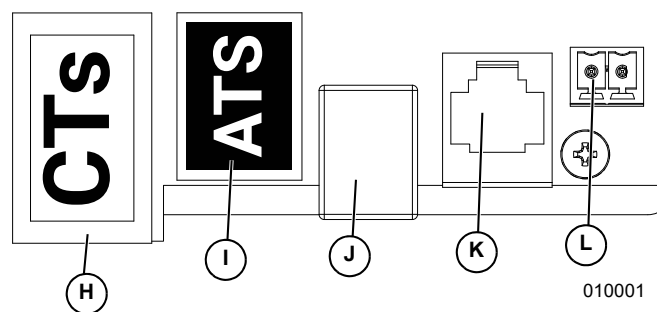
Figura 5-9. Puertos auxiliares
