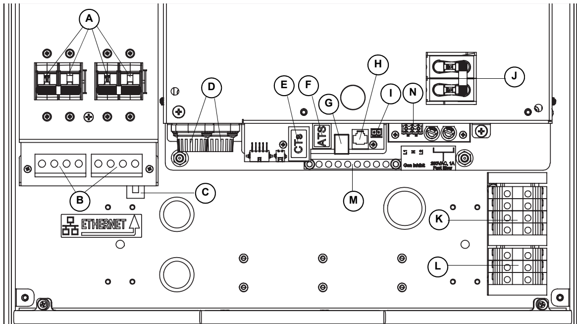
Figura 5-1. Compartimiento de cableado del inversor PWRcell
