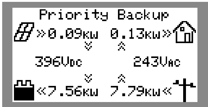
Figura 6-18. Modo actual
