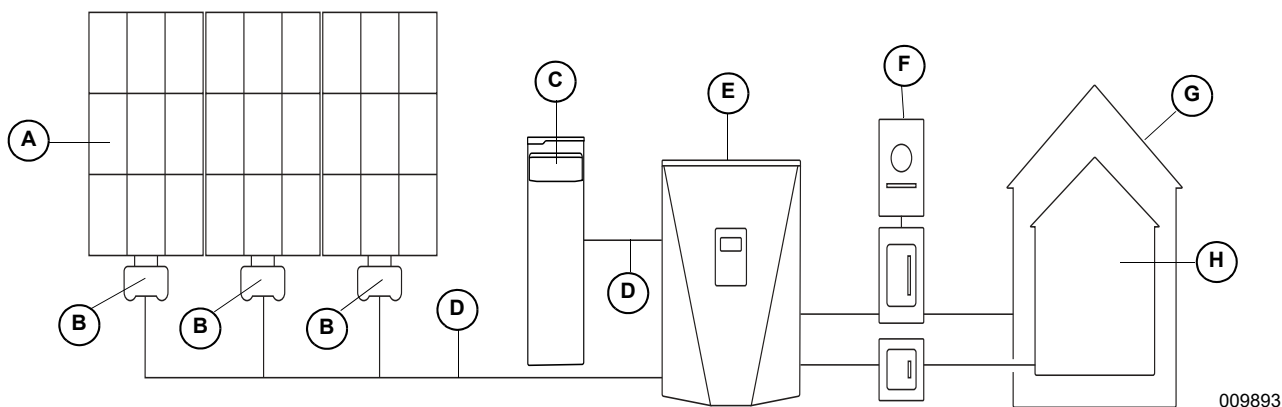
Figura 2-3. Ejemplo del sistema PWRcell de Generac
