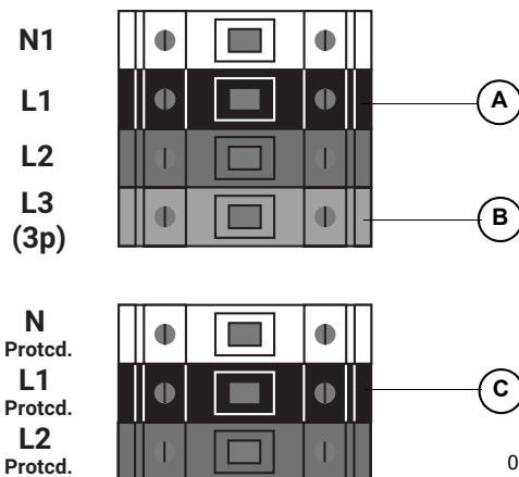
Figura 5-4. Terminales de cableado de CA
