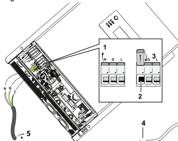
Figure 10 Acheminer et connecter les câbles d'entrée CA
