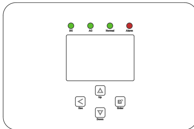
Figura 22: Interfaz de usuario e indicadores LED
