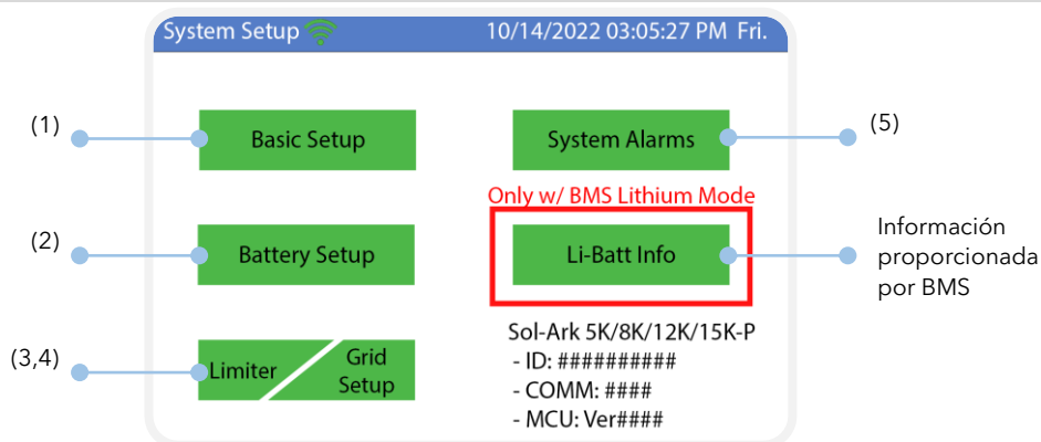
Figura 25: Pantalla de configuraciones
