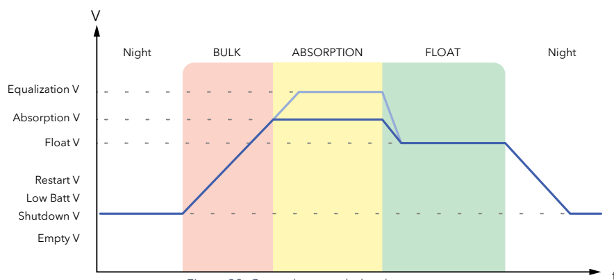
Figura 32: Curva de controlador de carga
