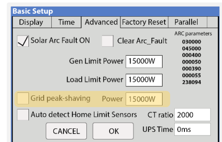
Figura 10: Parámetros de Grid peak-shaving
