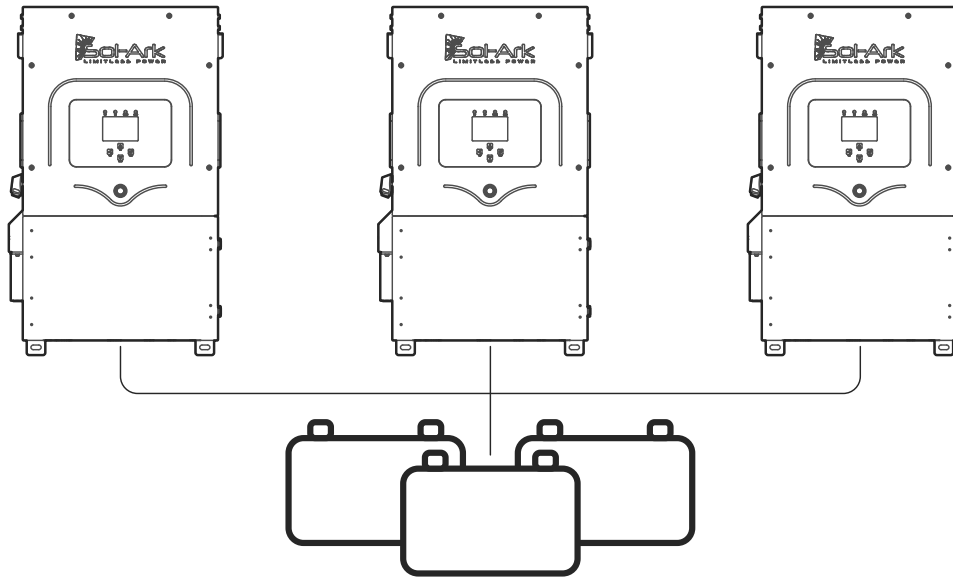
Figura 7: Único banco de baterías para inversores en paralelo
