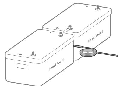
Figura 13: Sensor de temperatura para baterías de Ácido-Plomo
