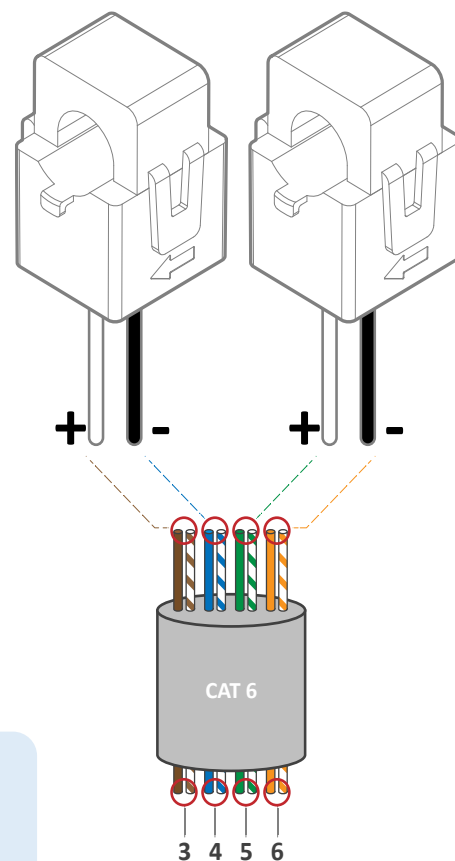
Figura 18: Extensión de sensores CT con cable CAT 6
