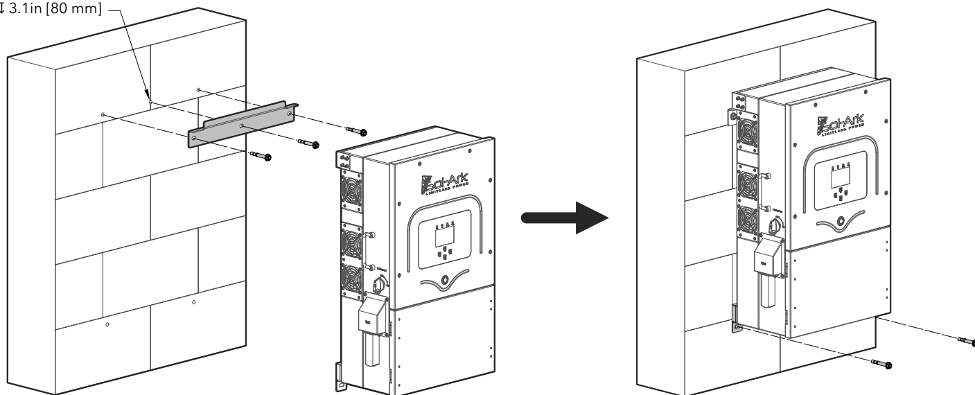
Figura 3: Montaje mural
