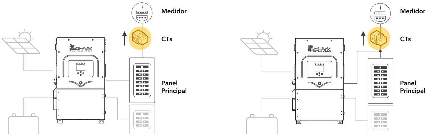
Figura 16: Instalación de CTs
