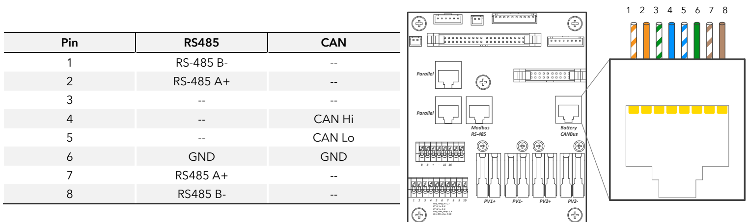
Figure 33: Configuración de puerto RJ45
