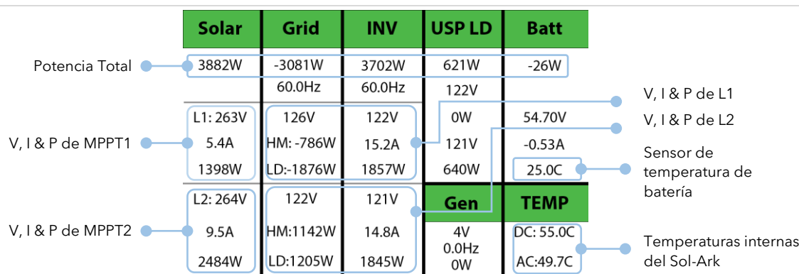
Figura 24: Pantalla de detalles
