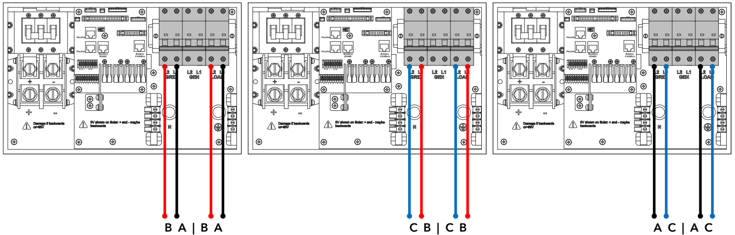
Figura 38: Ejemplo de secuencia de fases correcta
