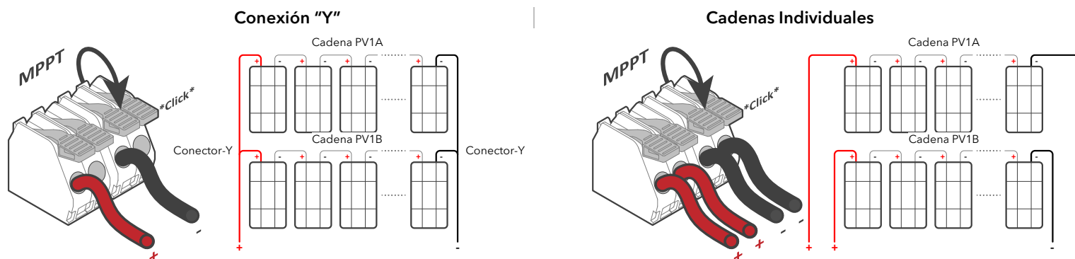
Figura 9: Cableado de MPPT y conexión de cadenas FV
