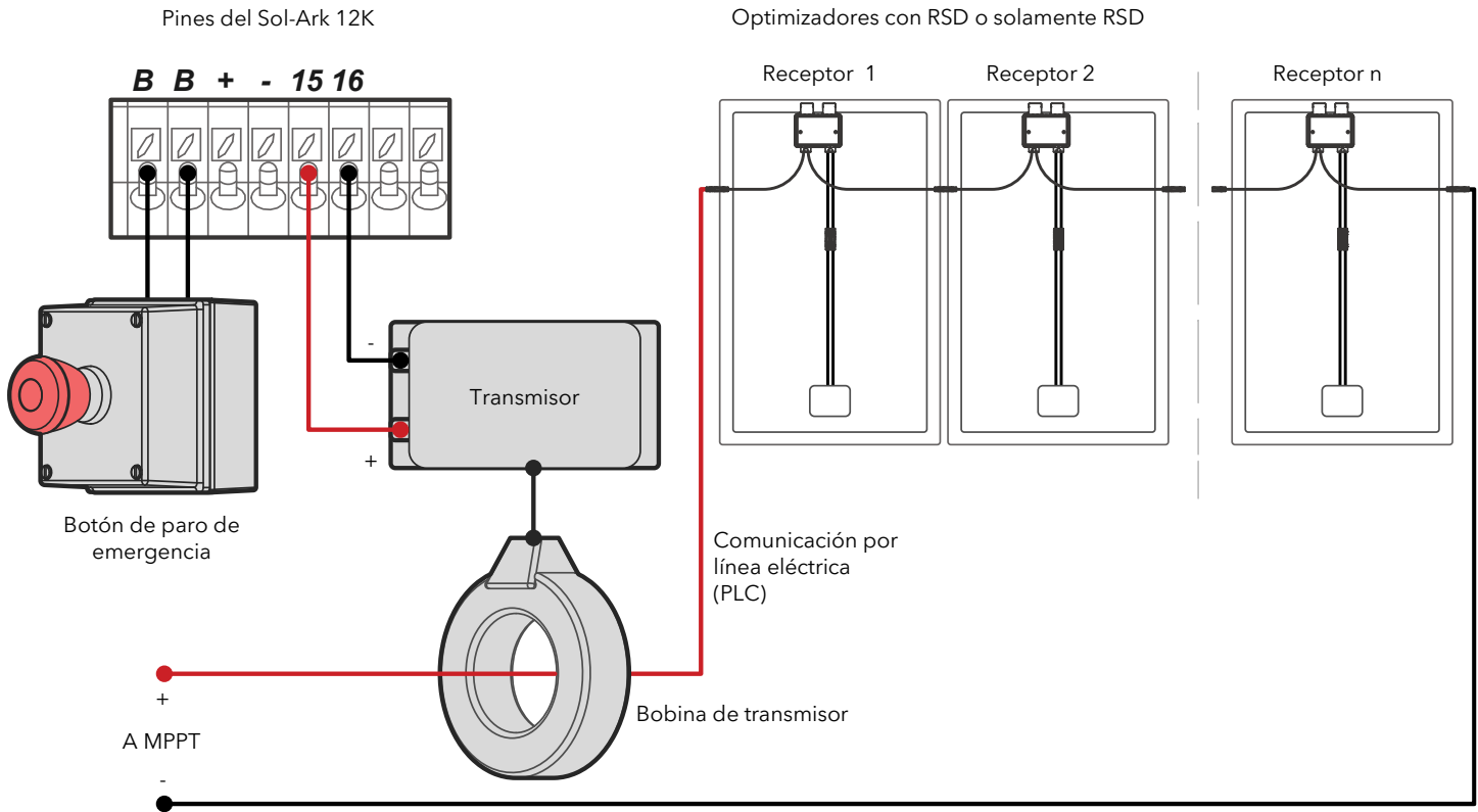
Figura 19: Paro de emergencia e instalación de RSD
