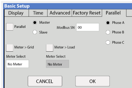
Figura 36: Pestaña de configuración de paralelo
